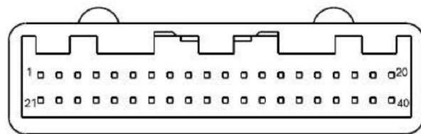
手动空调控制单元
